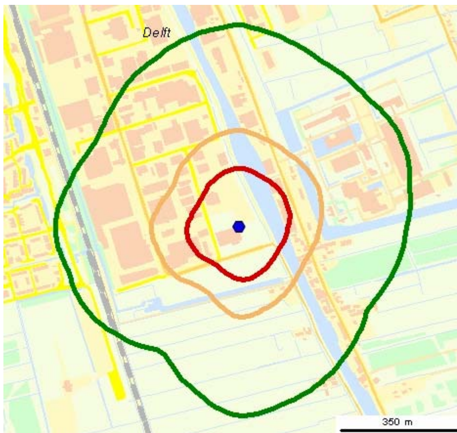
Afbeelding 9 Geurzones huisvuiloverslagstation
