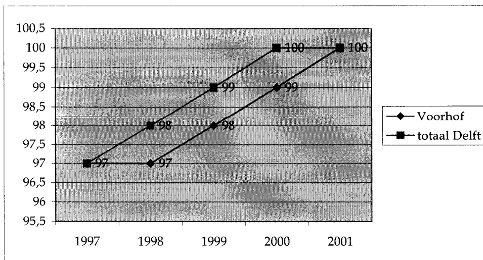
Figuur 4 Geïndexeerde groei van de bevolking in resp. heel Delft en Voorhof (periode 1997 – 2002, met 2001 als 100)
