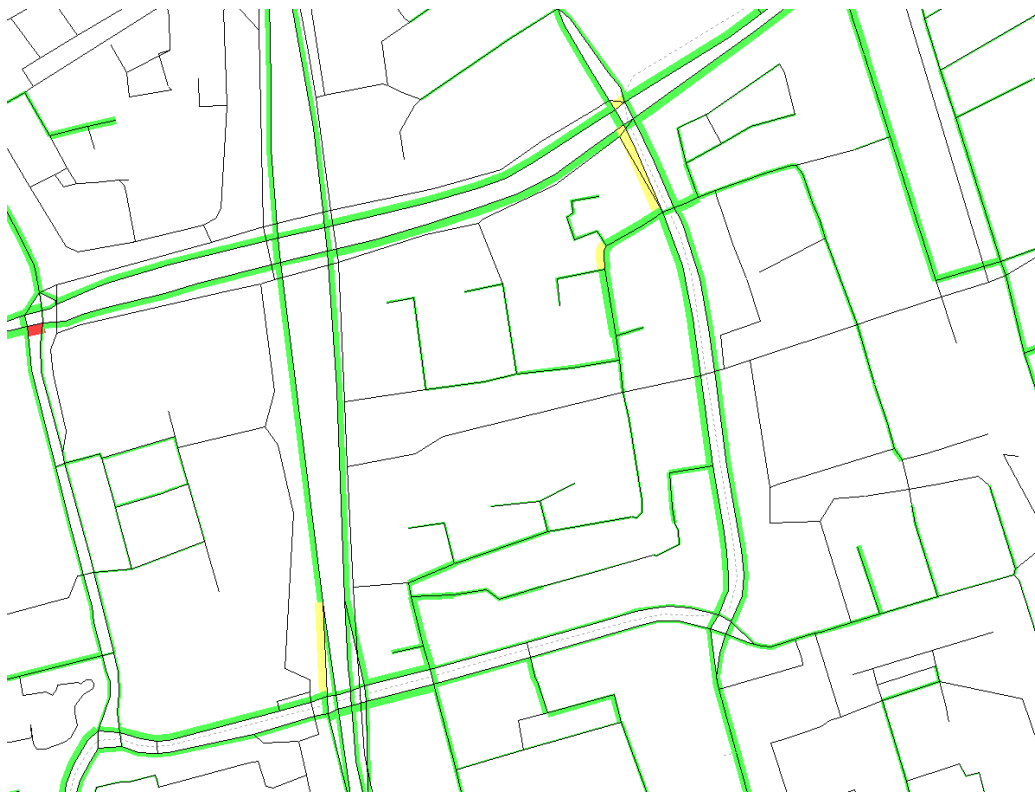
figuur 8: relatie intensiteit - capaciteit wegvakken
