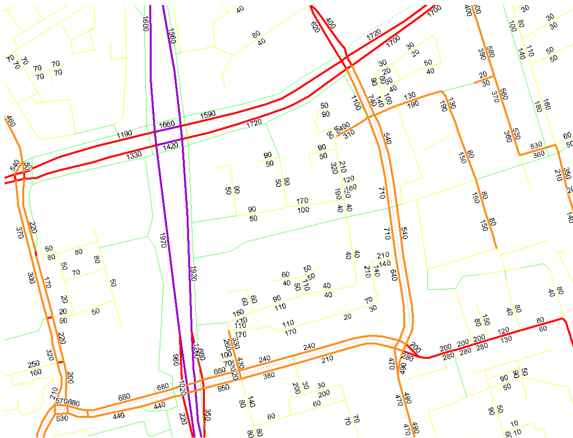
figuur 7: verkeersintensiteiten avondspitsuur
